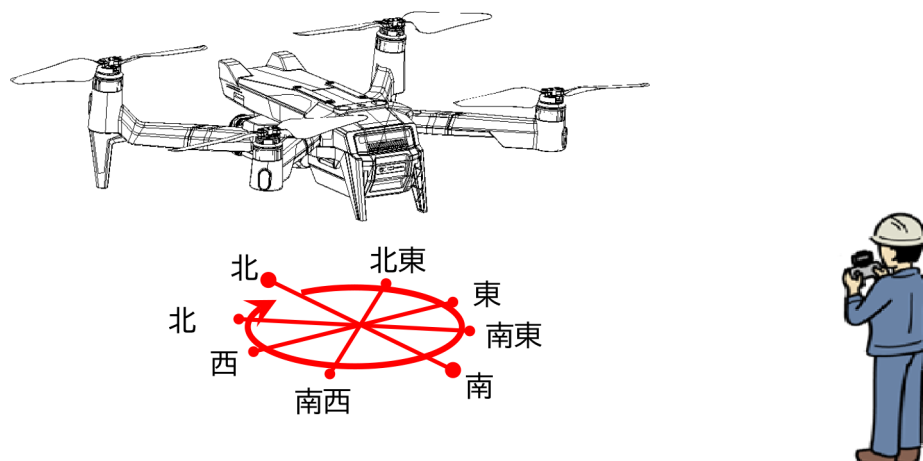
図 84 フルキャリブレーション：機首を8方位に向けてホバリング
